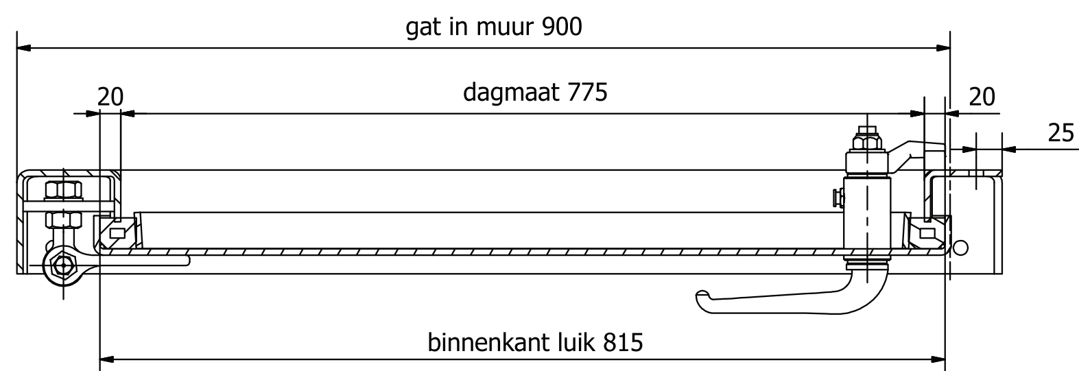
B-B ( 1 : 5 )
